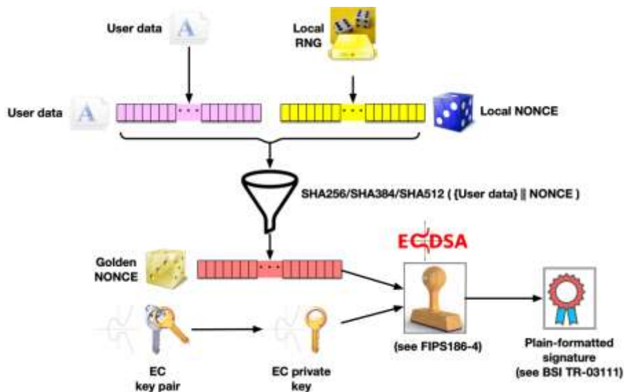
איור 5- מנגנון למניעת NONCE reuse
