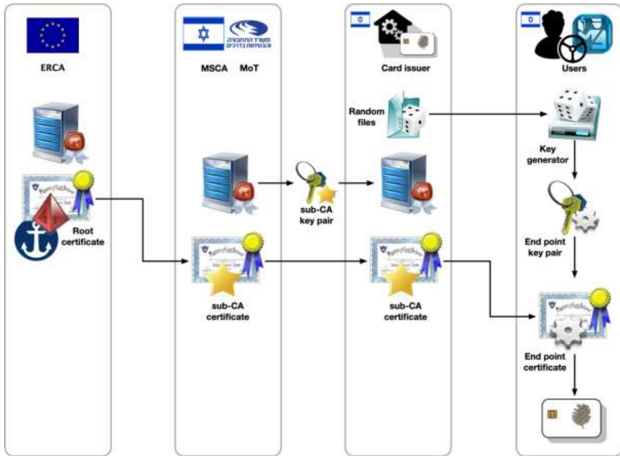
איור 3 - מדרג ה-PKI
