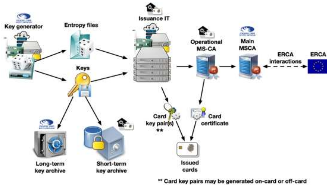
איור 2 - תשתיות מערך הצופן
