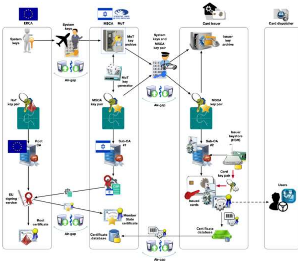
איור 4 - מערך הצופן - מבט על
